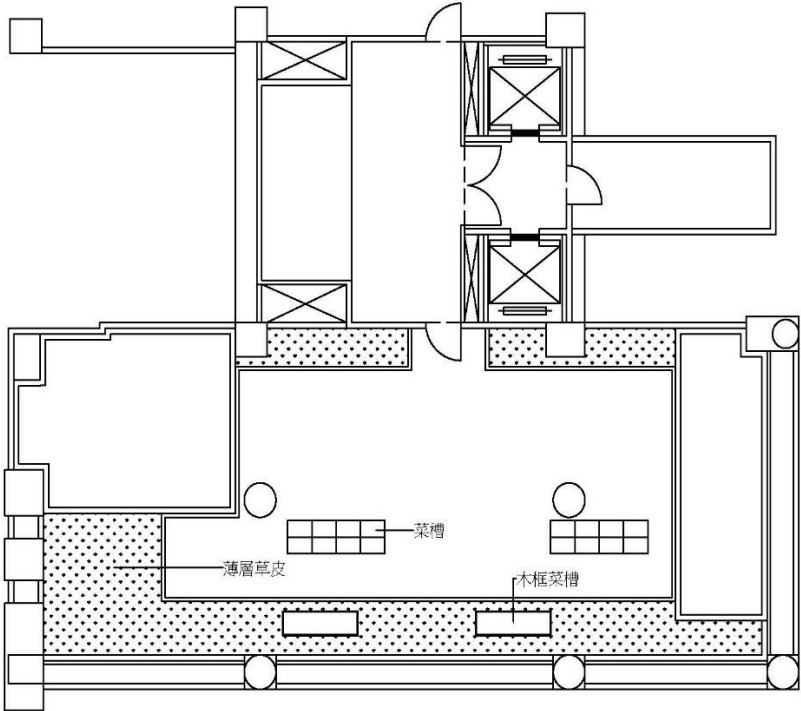
宏普光年領袖館社區 A 棟平面圖
