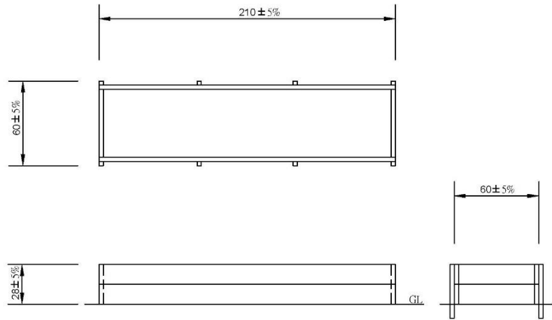
菜槽及南方松木框菜槽設計圖 (尺寸誤差值正負 5%內)
